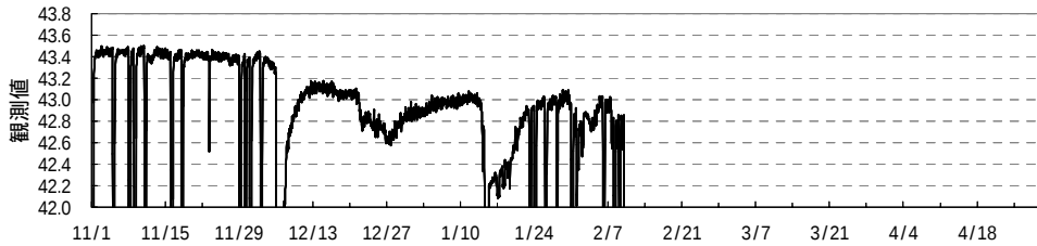
出雲湯村温泉 水温( )
