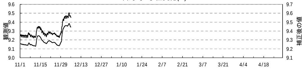
日野町 水位変化(m)
