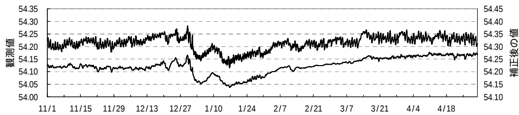
鳥取温泉 水温( )
