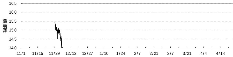
日野町 水温( )
