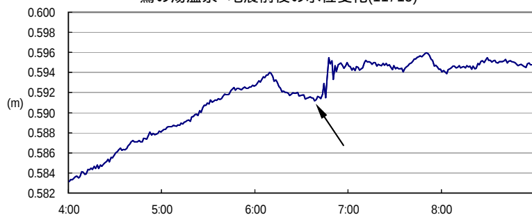
鷺の湯温泉 地震前後の水位変化(11/15)
