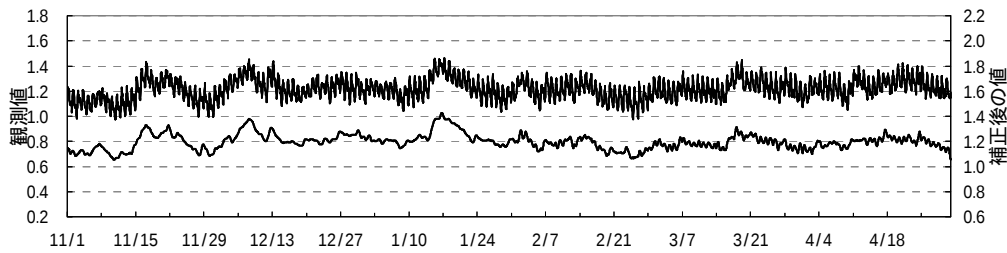
岩井温泉 水位変化(m)
