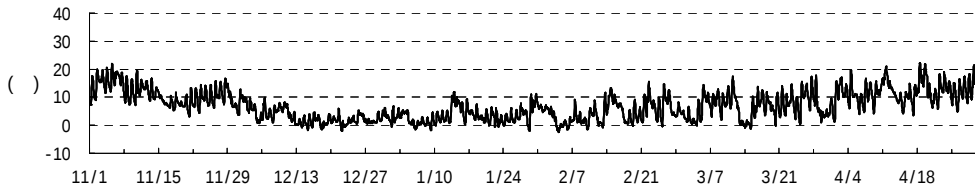
鳥取市 気温
