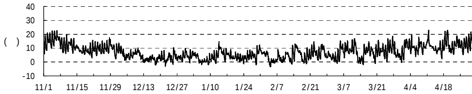
松江市 気温
