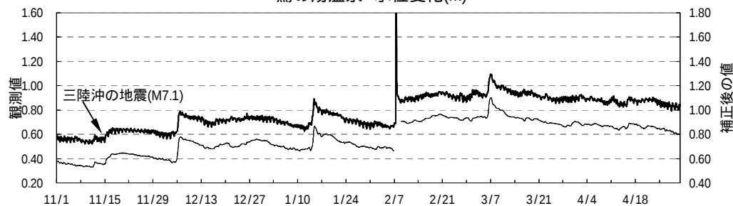
鷺の湯温泉 水位変化(m)
