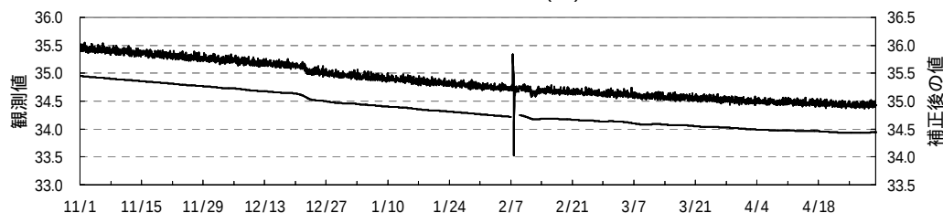
鷺の湯温泉 水温( )
