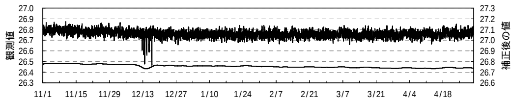
鹿野温泉 水温( )
