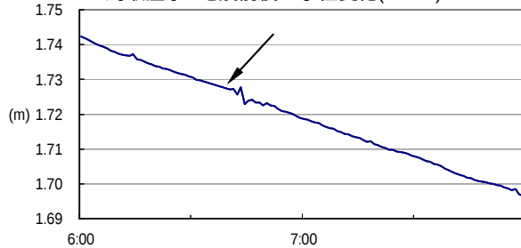
鳥取温泉 地震前後の水位変化(11/15)
