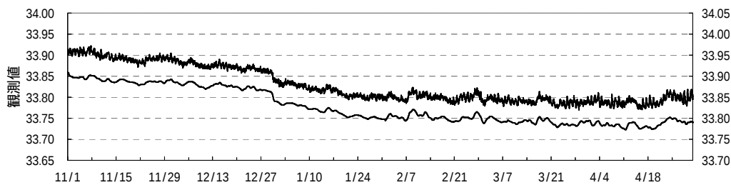
湯谷温泉 水温( )
