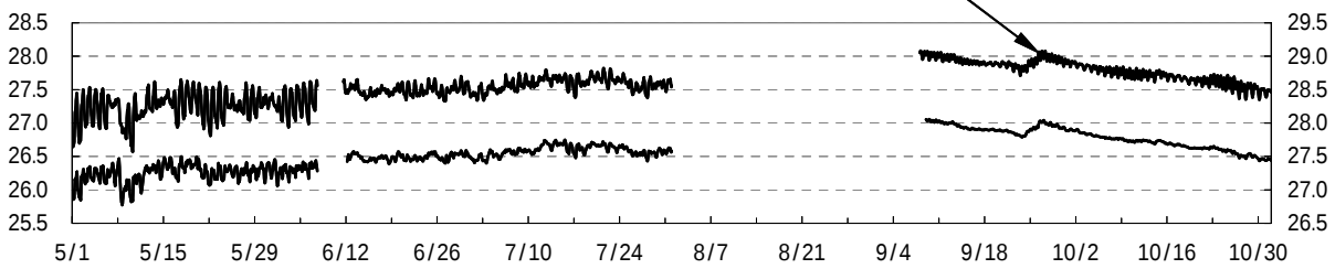
奥津温泉 水温( ) 十勝沖地震(M8.0)
