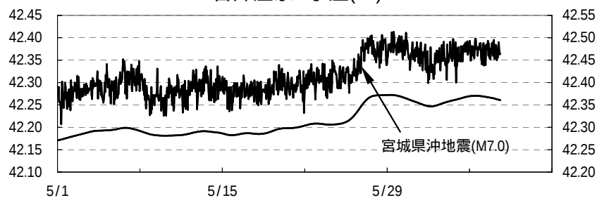
岩井温泉 水温( )
