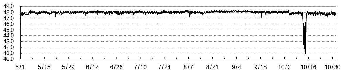
湯原温泉 水温( )
