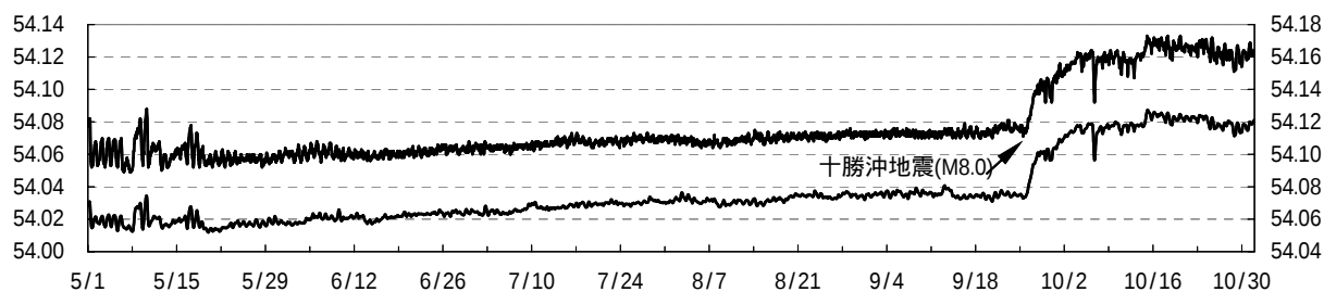
鳥取温泉 水温(°C)
