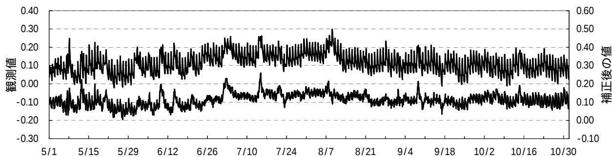
鳥取温泉 水位変化(m)
