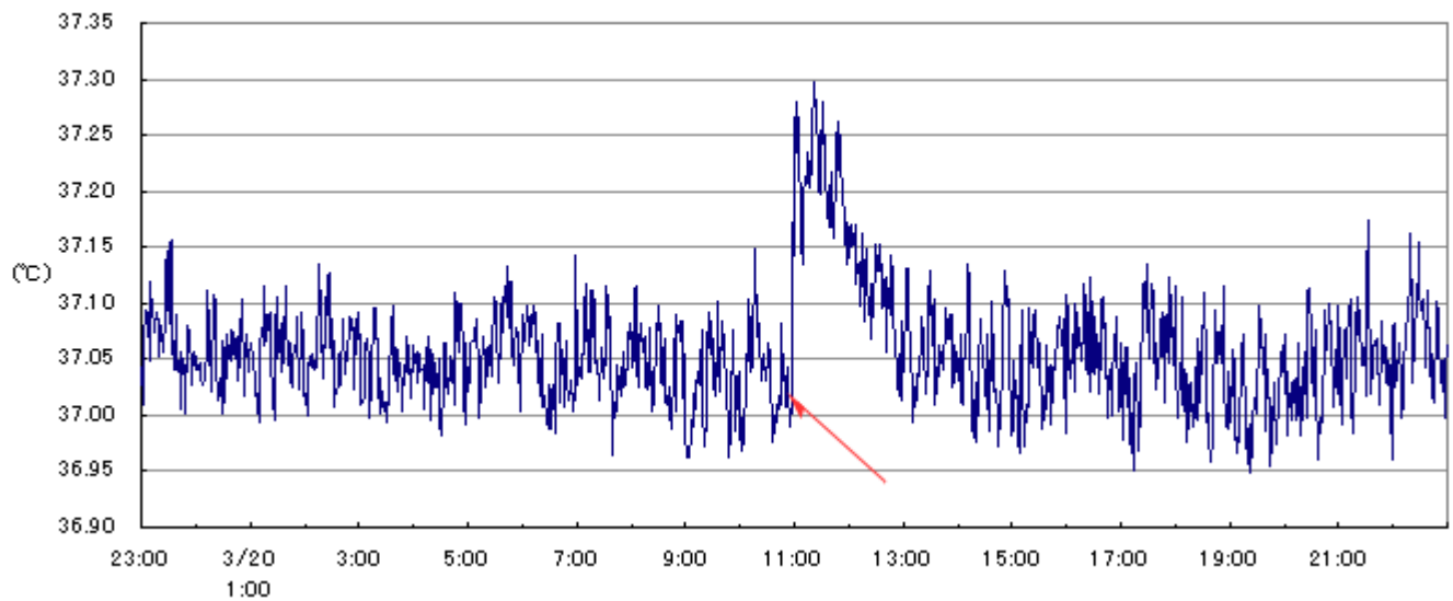
鷺の湯温泉 地震前後の水温変化
