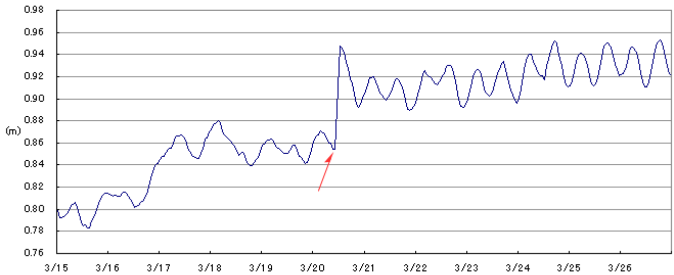
鷺の湯温泉 地震前後の水位変化(3/15~3/26)
