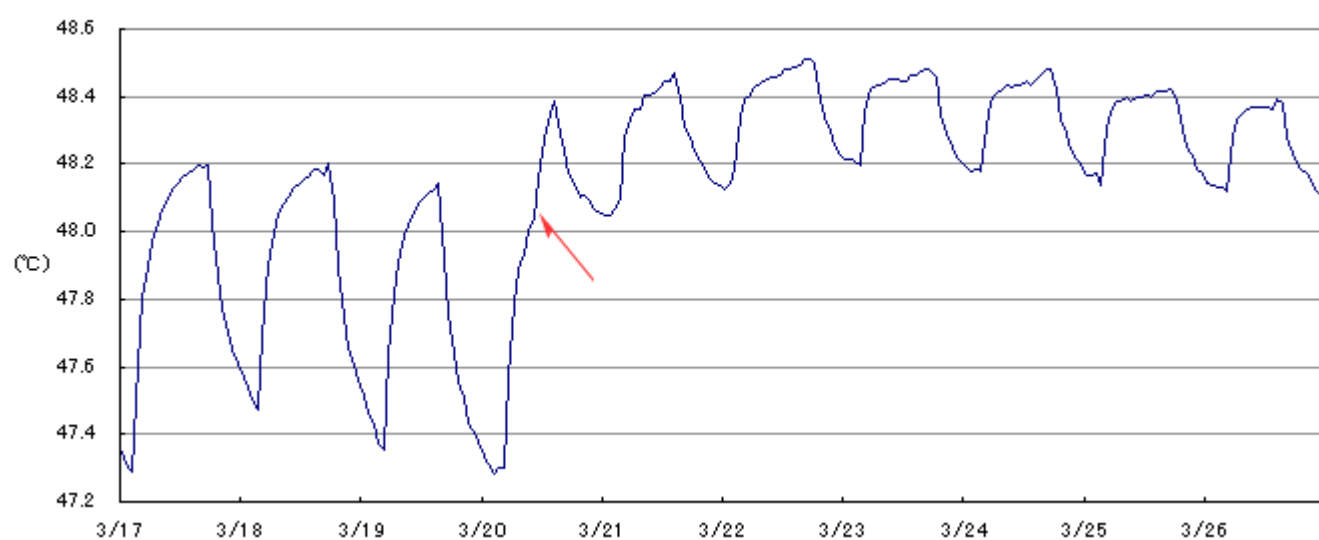
吉岡温泉 地震前後の水温変化(3/17~3/26)
